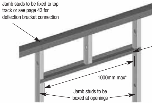
Fig. 1 Door Opening
