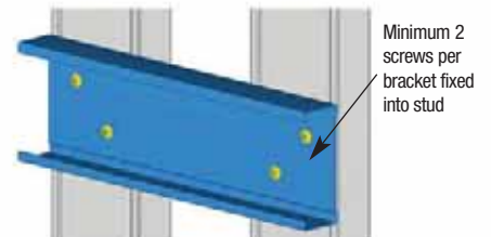
Fig. 5 Steel stud bridging
