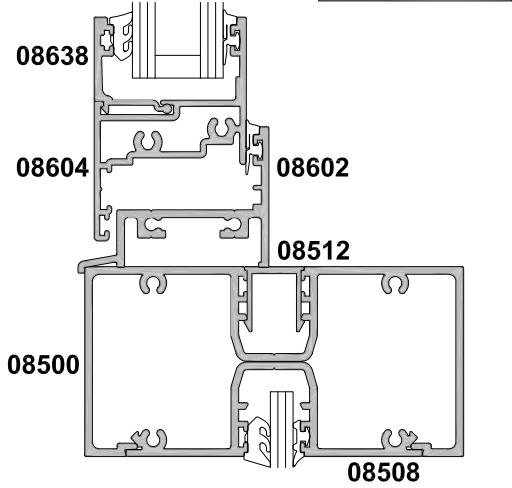
SECTION D-D
