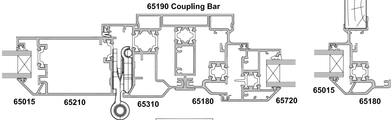
SECTION A-A OPEN OUT DOOR
