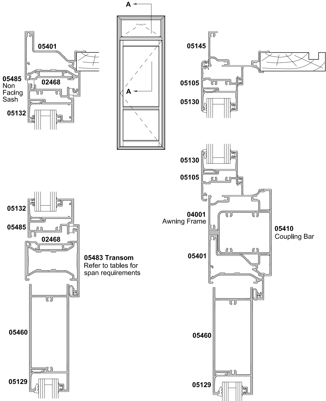
SECTION A-A
