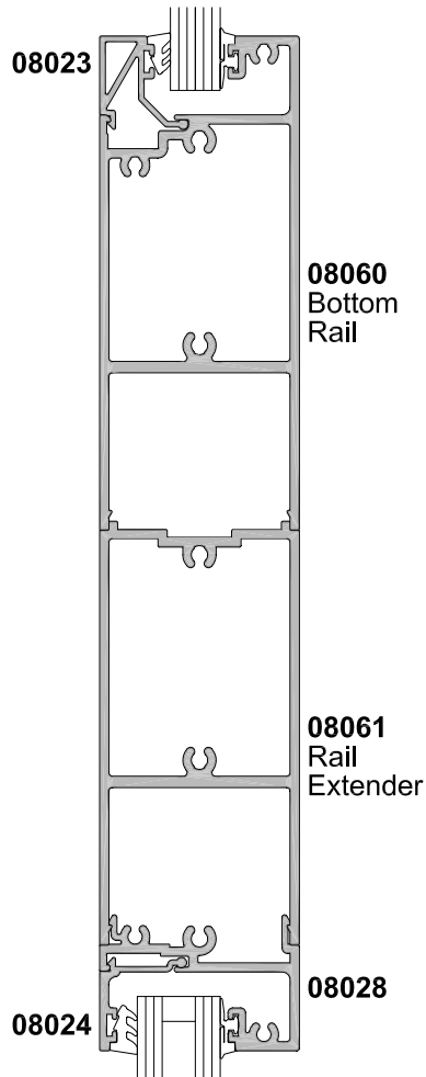
SECTION A-A
