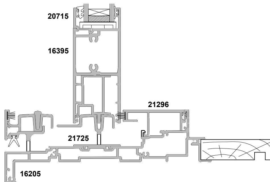
SECTION A-A
