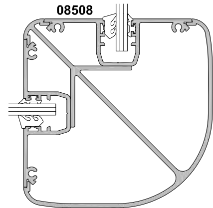
08567 90° Corner Post
