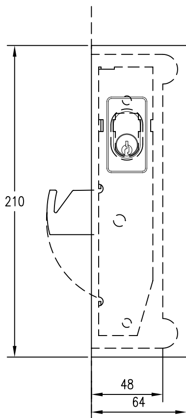
ELEVATION
