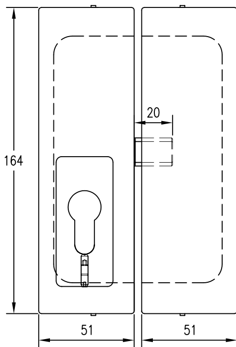
ELEVATION
