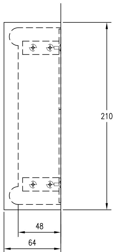
ELEVATION
