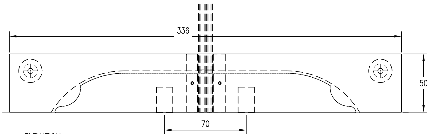
ELEVATION
