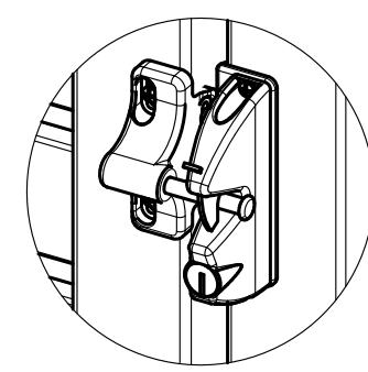
LOKKLATCH ON PED GATE 1:4
