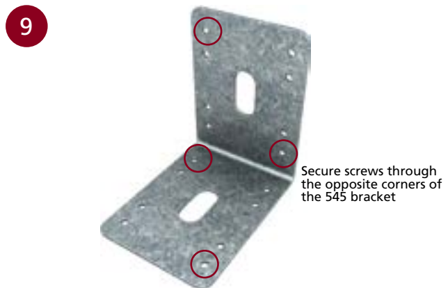
■ 545 BRACKET
