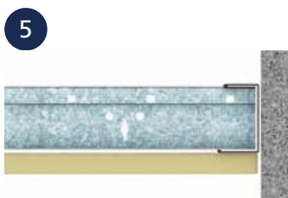
5 ■ PERIMETER DETAIL: XD6
