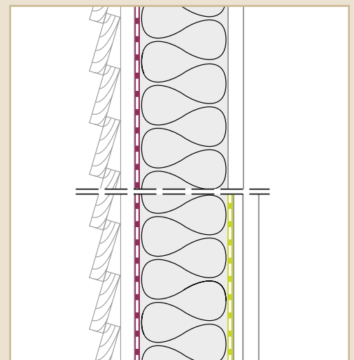
Fig. 47. Setup B
