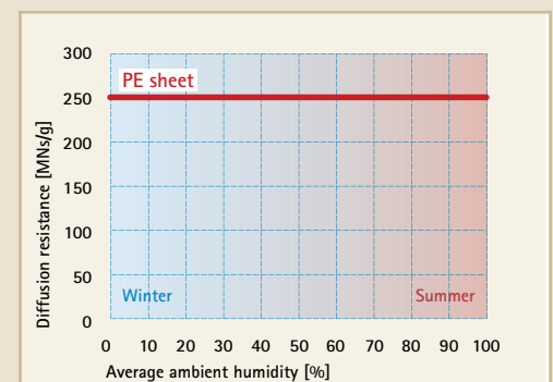
Fig. 28. Vapour diffusion resistance characteristics: Vapour barrier PE sheet
