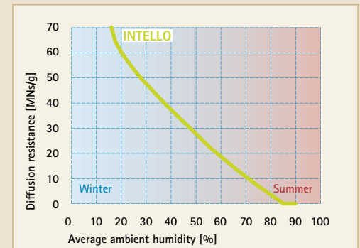
Fig. 27. Vapour diffusion resistance characteristics: pro clima INTELLO airtightness membrane
