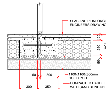
THERMAL BREAK
