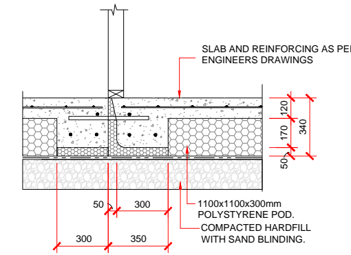
THERMAL BREAK
