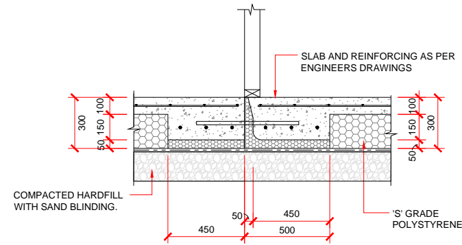
THERMAL BREAK
