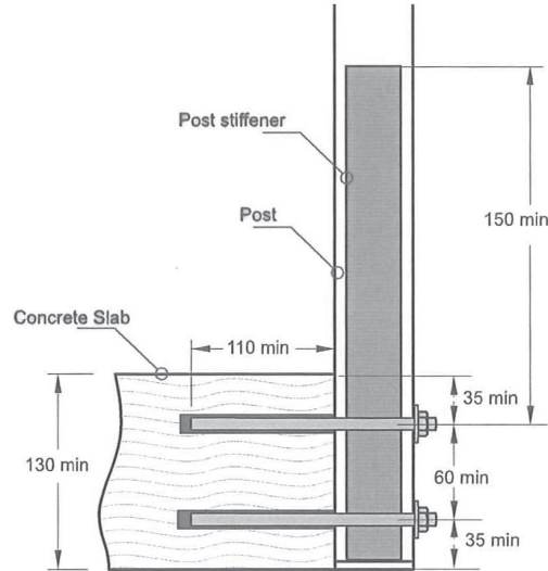
Bolt setout
