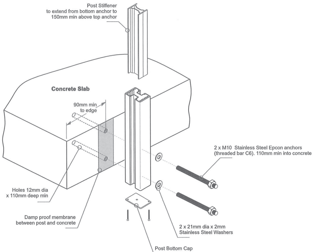
Bolt setout
