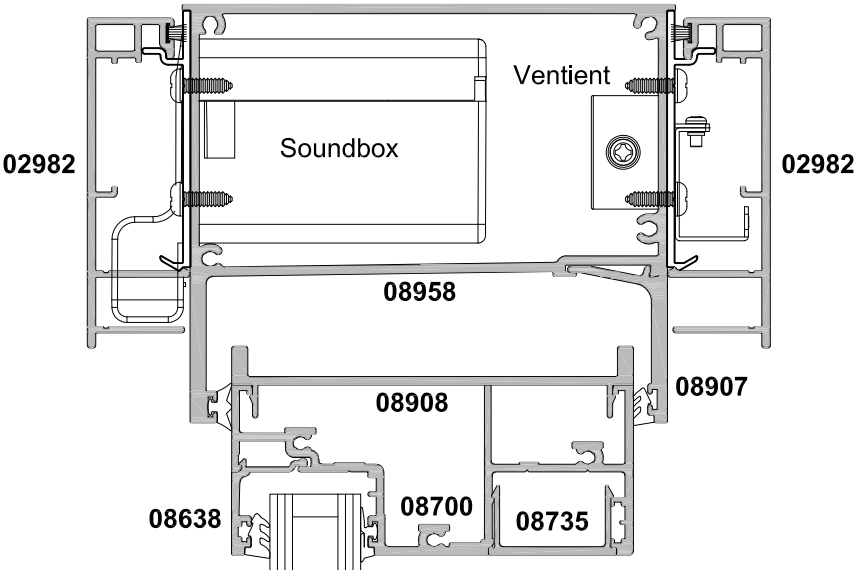
106MM VENTIENT FRAME
