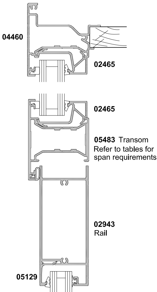
SECTION A-A
