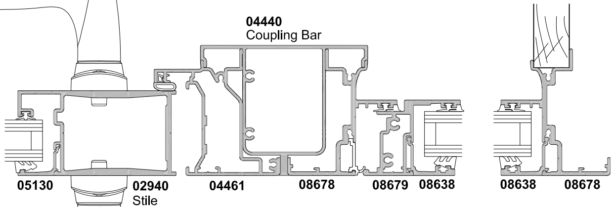
SECTION B-B OPEN OUT DOOR
