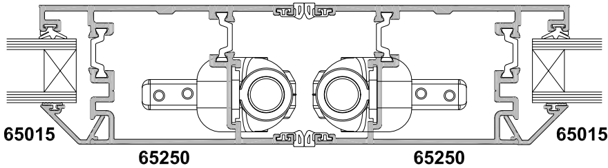
SECTION A-A
