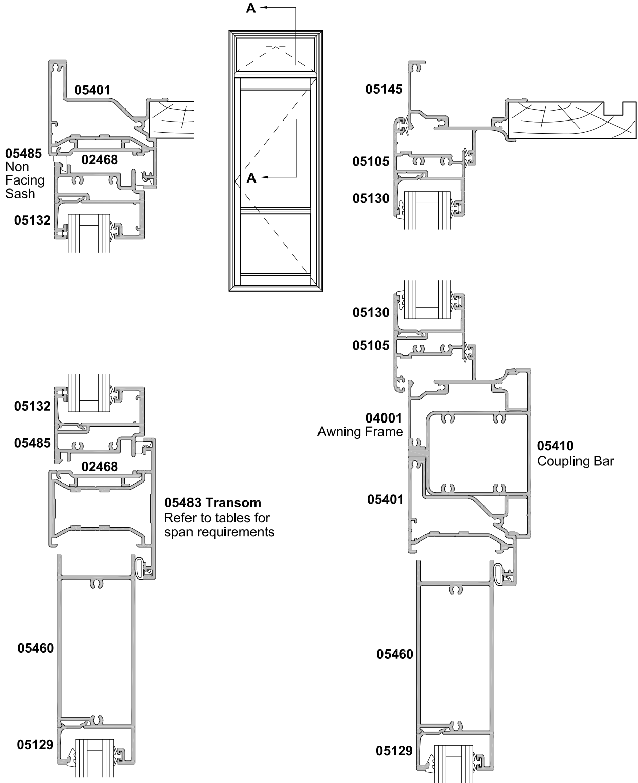
SECTION A-A
