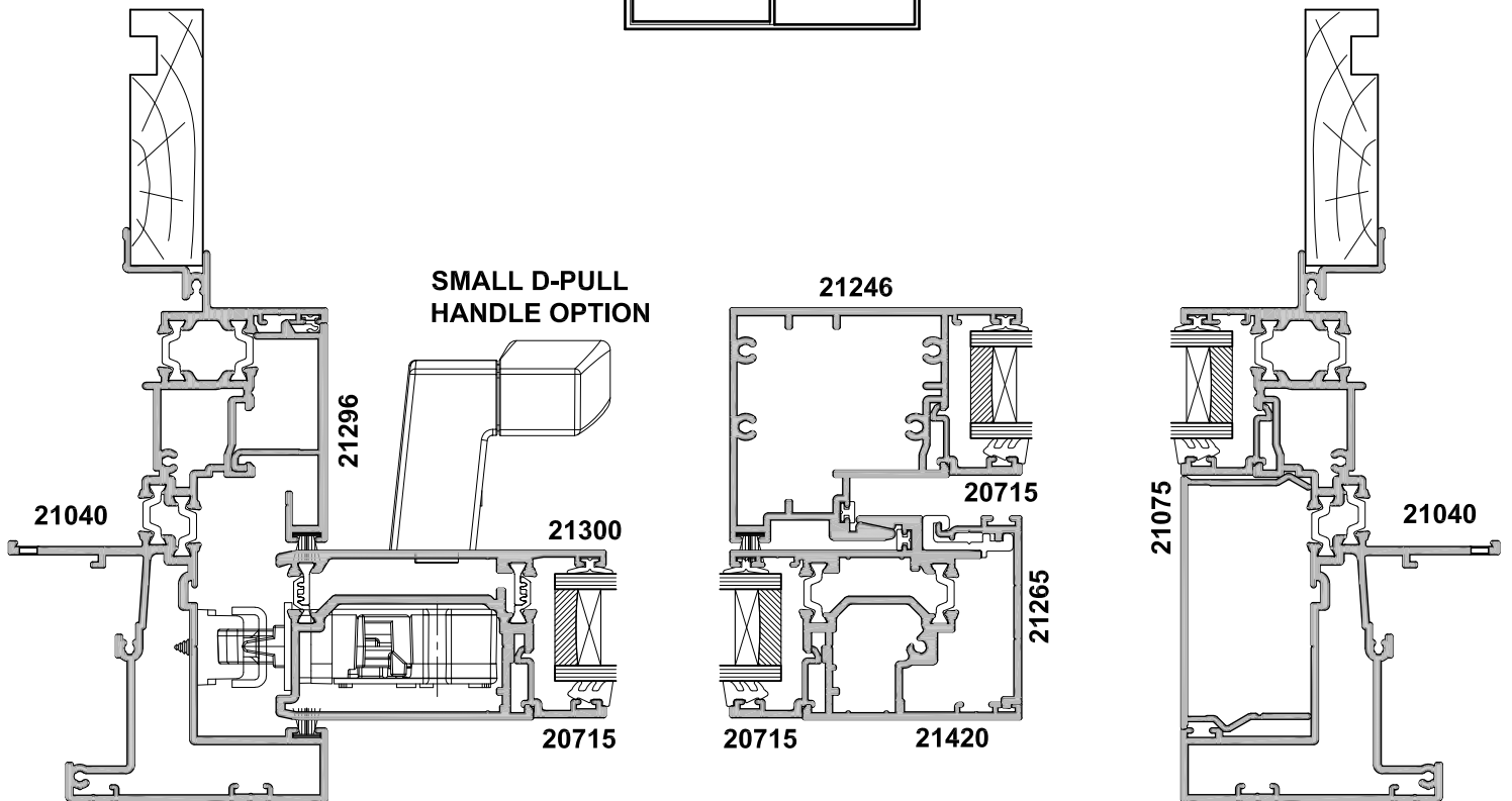
SECTION A-A
