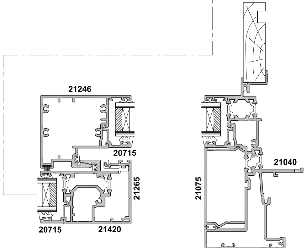
SECTION A-A
