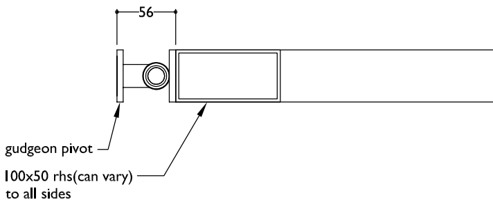
PLAN SECTION - END PIVOT(STANDARD)
