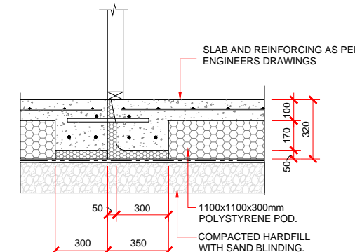
THERMAL BREAK
